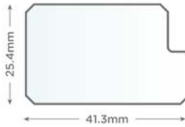
41.3mm Rebate Stile
