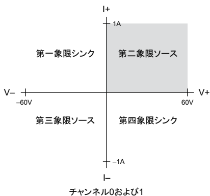
図 1. NI 4112 象限図
