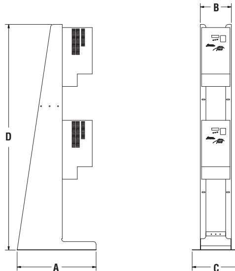
CS-VMP-2
