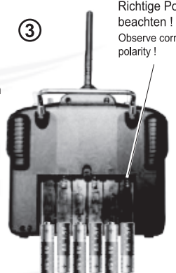
6 X 1,5V AA Batterien 6 X 1.5V AA batteries
