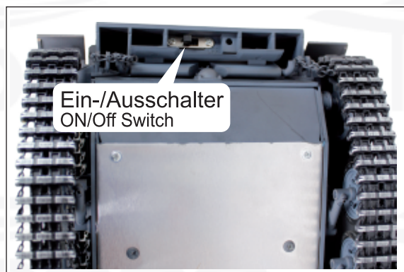
UNTERSEITE PANZER BOTTOM OF TANK
