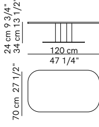
Tavolino 70 x 120 Small table 70 x 120
