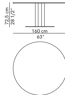
Tavolo Ø 160 Table Ø 160
