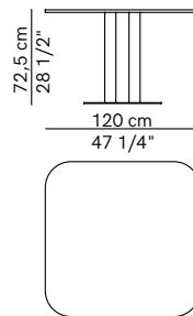
Tavolo 120 x 120 Table 120 x 120
