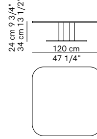
Tavolino 120 x 120 Small table 120 x 120
