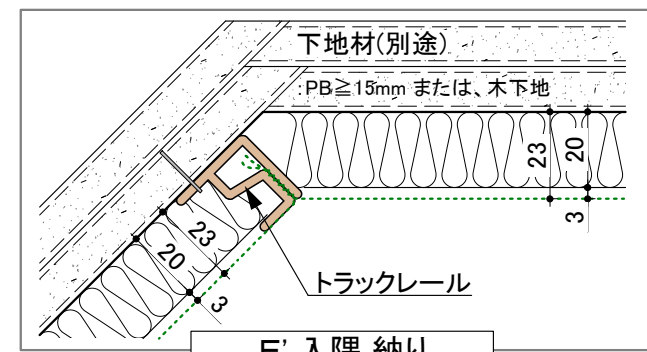
E' 入隅 納り
