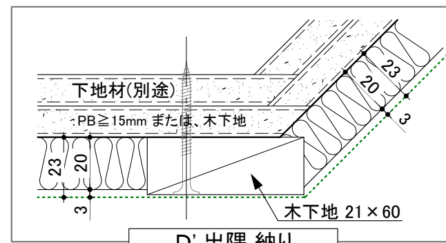
D' 出隅 納り
