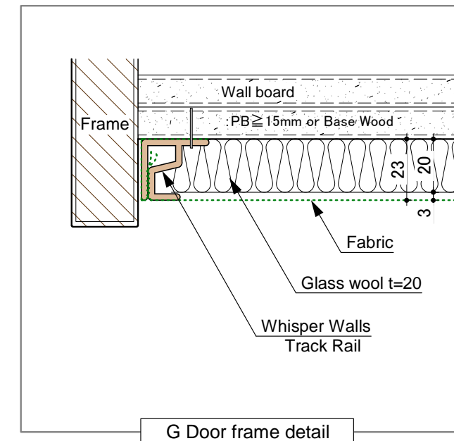
G Door frame detail
