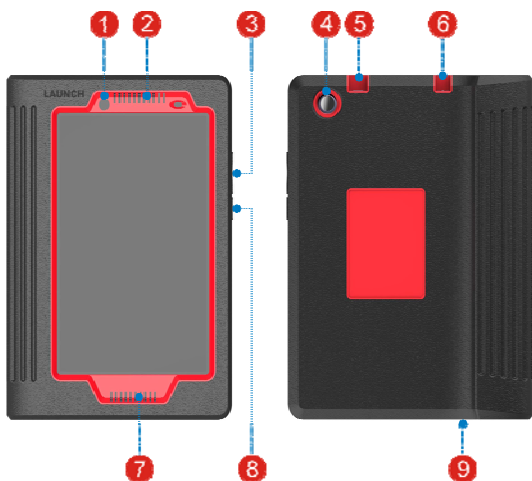
Fig. 1-2 X-431 PRO handset
