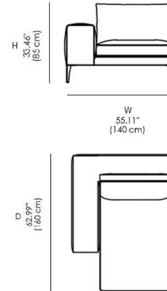
Side Element 140 L SX/DX
