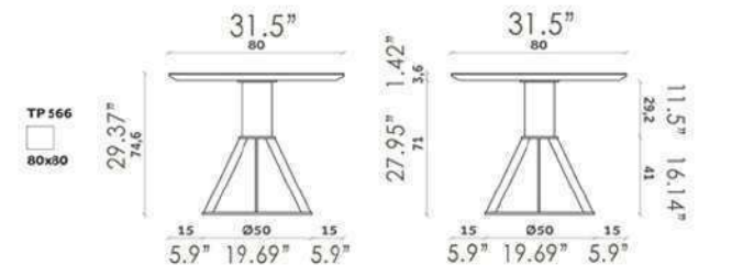
GERONIMO Table Design Paolo Cappello PIANI FISSI CERAMICA FIXED CERAMIC TOPS
