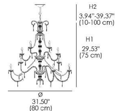
117 Chandelier (117/6+3)
