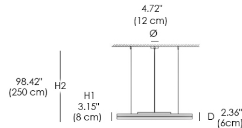
Lite Hole S90
