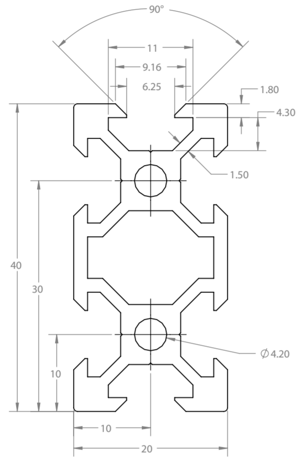
V-Slot 20X40 Linear Rail
