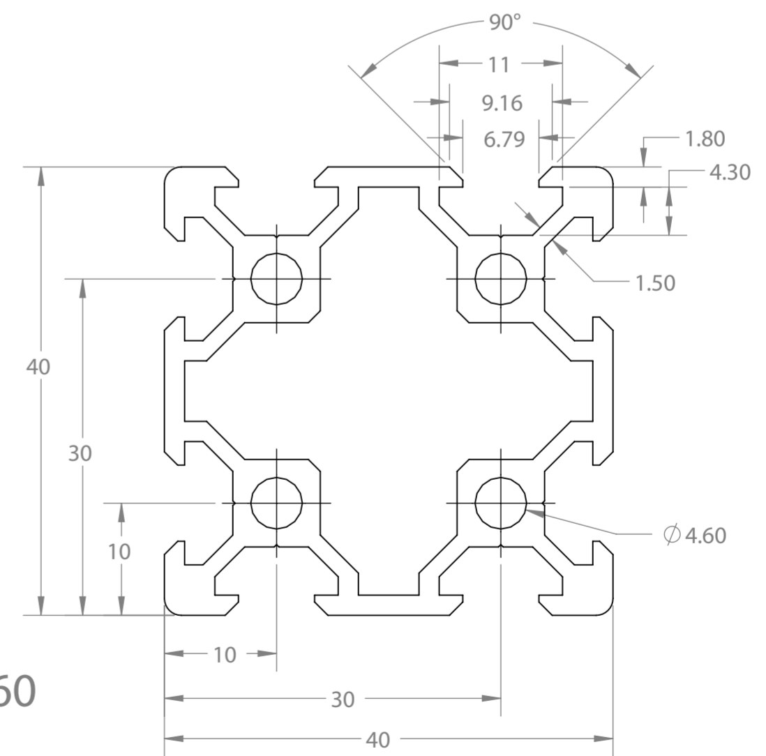
V-Slot 40X40 Linear Rail
