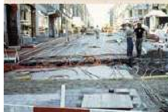
Arbeider med gatevarme i Karl Johans gate i Oslo i 1976.
