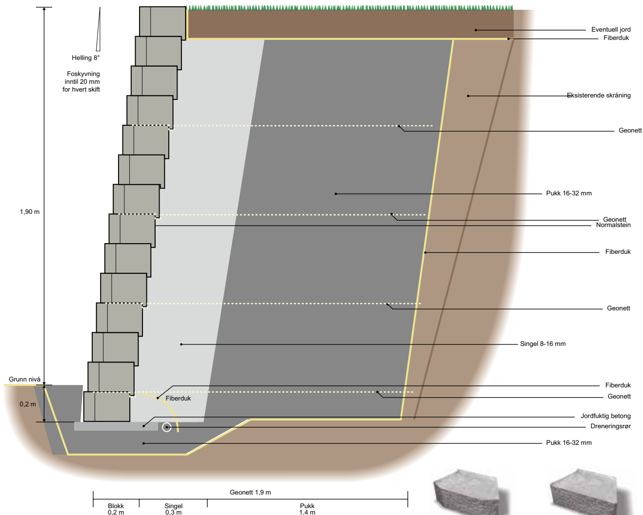
Bilde 5. Snittegning av Megastone 150 rundhugd 385 x 220 x 150 og retthugd 400 x 220 x 150.
