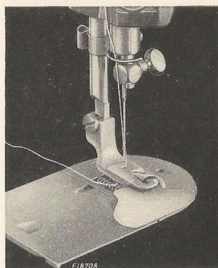
FIG. 195. THE FLANGE HEMMER
