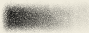
Dusty Shader
