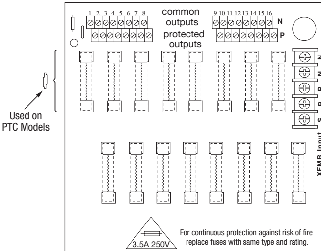
Fig. 4 - PD16W/PD16WCB
