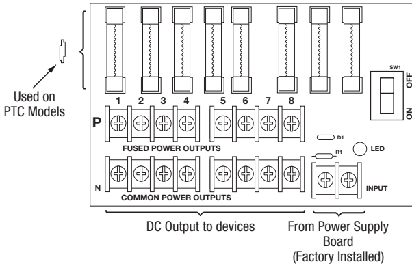
Fig. 3 - PD8/PD8CB
