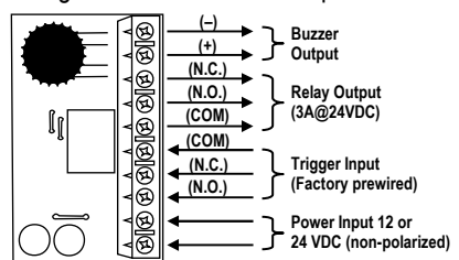
Fig. 10 – Timer Module Top View
