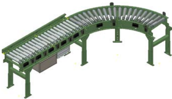
E24EZ / E24EZC
