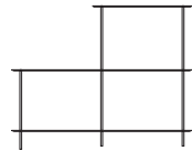
Mid 1.5 W 1180 D 370 H 561/950
