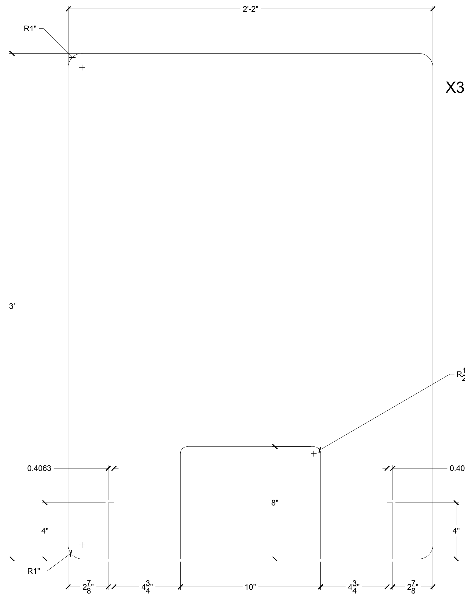
SNEEZE GUARD - PLEXI LAYOUT SCALE: 3" = 1'-0"
