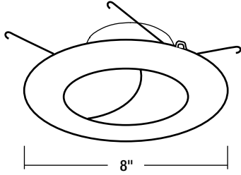
Trim OD: 8"
