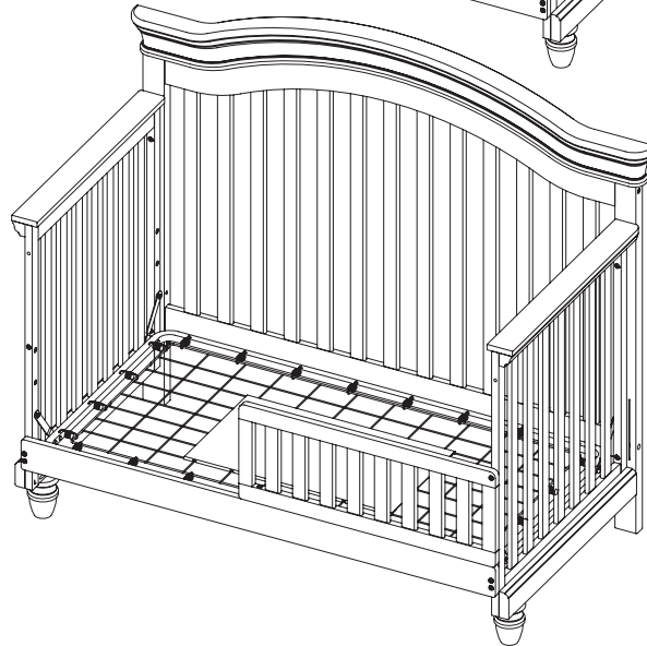
FIG. 1B RIGHT GUARD INSTALLATION FIG. 1B INSTALLATION DU GARDE-CORPS À DROITE FIGURA 1A INSTALACION DEL RIEL PROTECTOR LADO DERECHO
