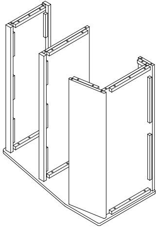
From Step 1 del paso 1
