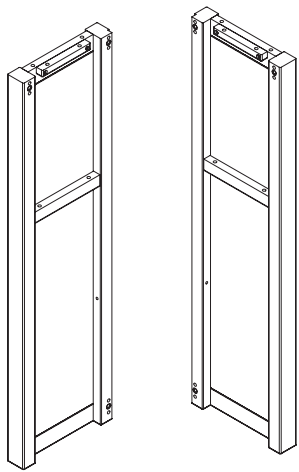
A. Left Side x1 Côté gauche Lado izquierdo Part# 25559 B. Right Side x1 Côté droit Lado derecho Part# 25560
