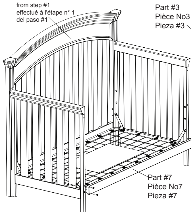
#6 - (2) M6 x 35mm BOLT (2) BOULONS M6 x 35mm (2) PERNOS M6 x 35mm
