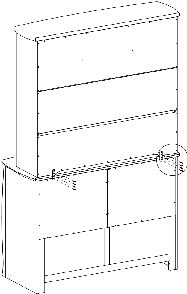
KK. Metal Plate x2 Plaque de métal Bandejas Metálicas
