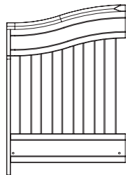
C. - (1) Right Crib Side (1) Panneau de Droite du Lit de Bébé (1) Lado derecho de la Cuna 23848
