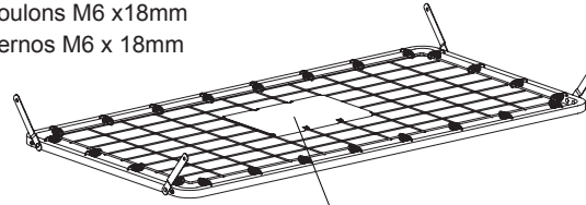
#8 - (1) Mattress Support (1) Support de Matelas (1) Soporte para el Colchón
