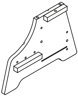
A. Left Side x1 Part #21846
