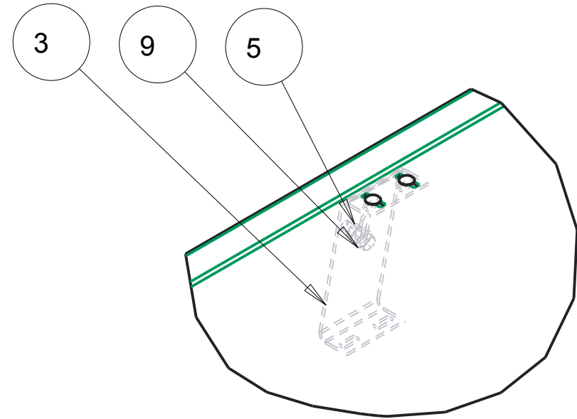
DETAIL E SCALE 0.200
