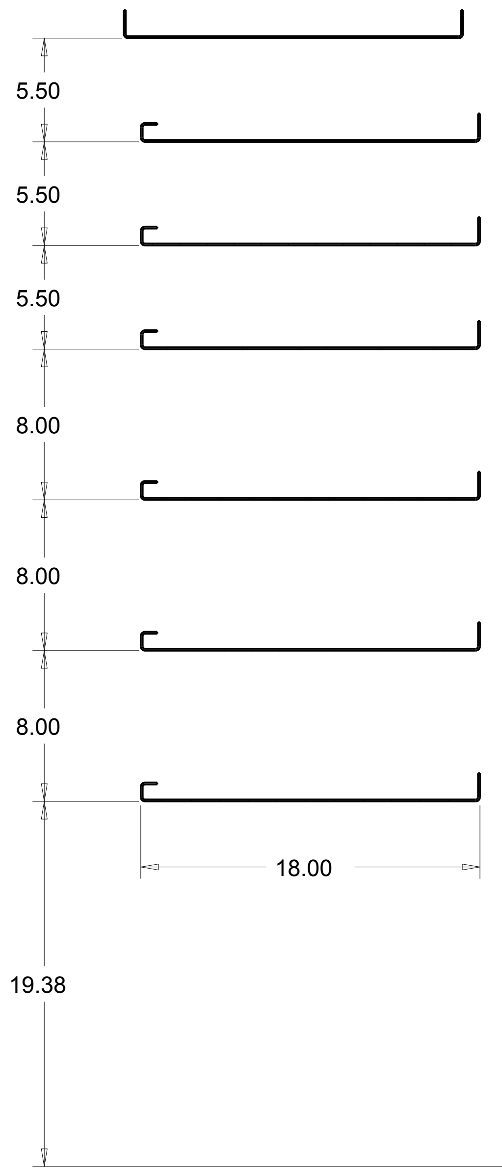
SECTION A-A
