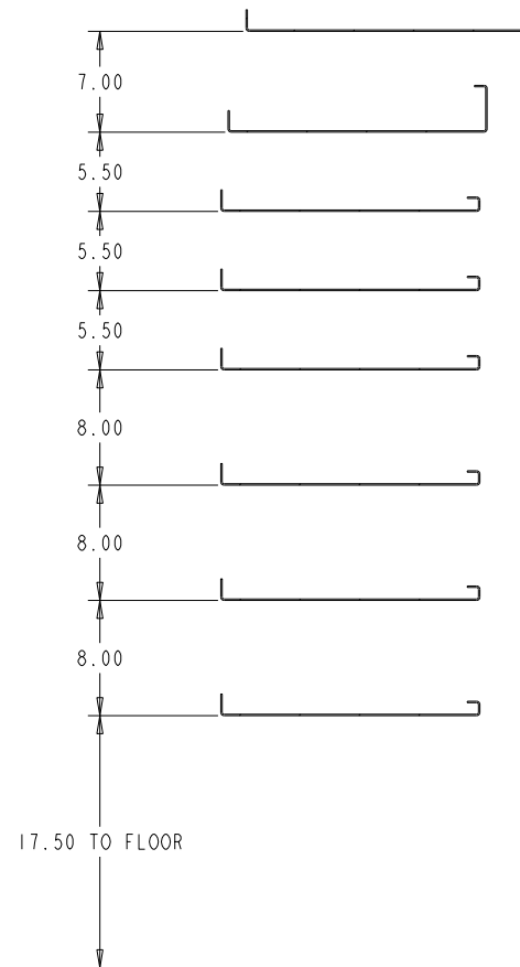
SECTION C-C SCALE 0.150
