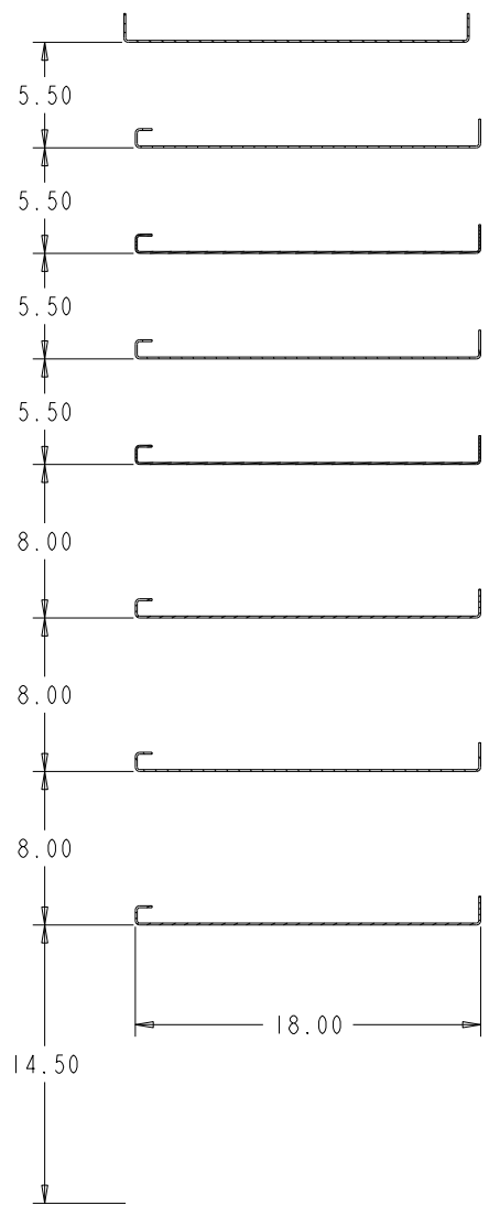
SECTION A-A
