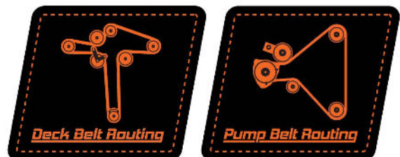
491-0169-00 RZ-Pro Model Decal
