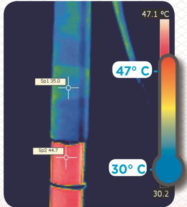
· Pipa de agua caliente con y sin THERMO-BAND® (Vista Infrarrojo)
