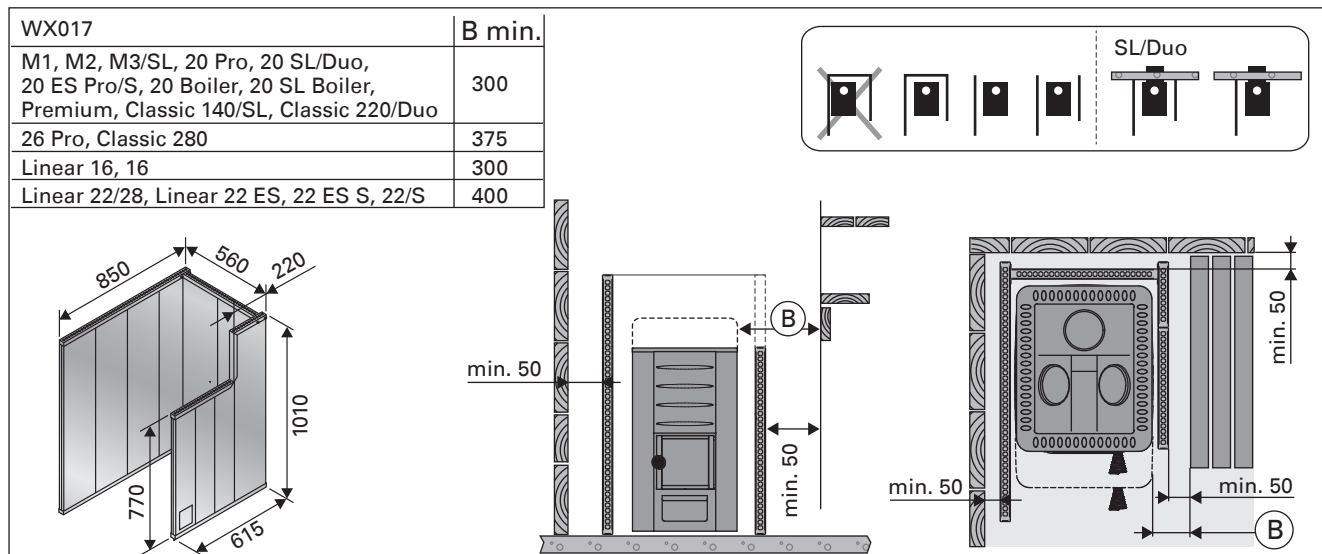
Рисунок 7. Безопасные расстояния (все размеры приведены в миллиметрах) Joonis 7. Ohutuskaugused (kõik mõõtmised millimeetrites)
