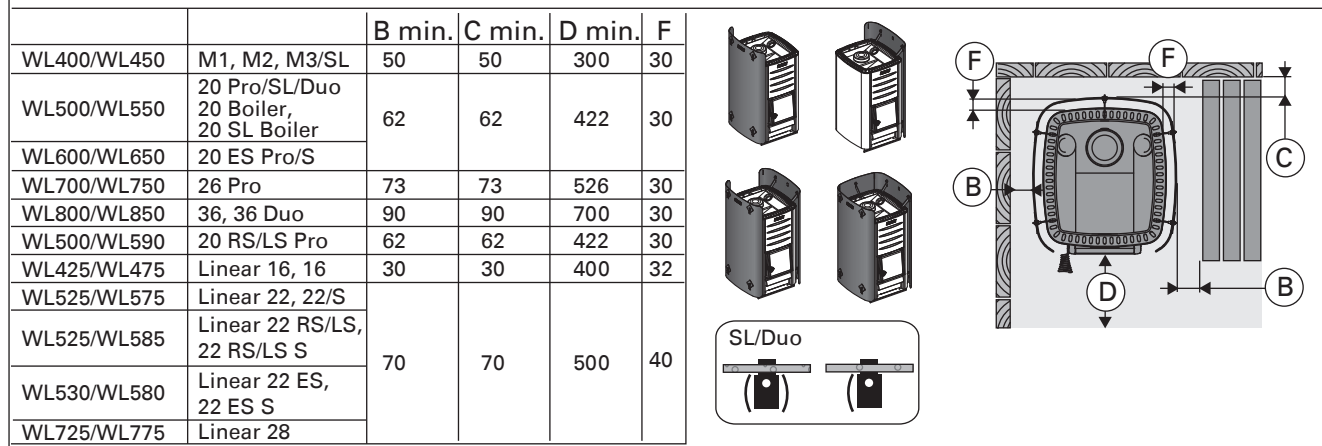
Рисунок 8. Безопасные расстояния с защитными ограждениями (все размеры приведены в миллиметрах) Joonis 8. Ohutuskaugus koos kaitseseinaga (kõik mõõtmised millimeetrites)
