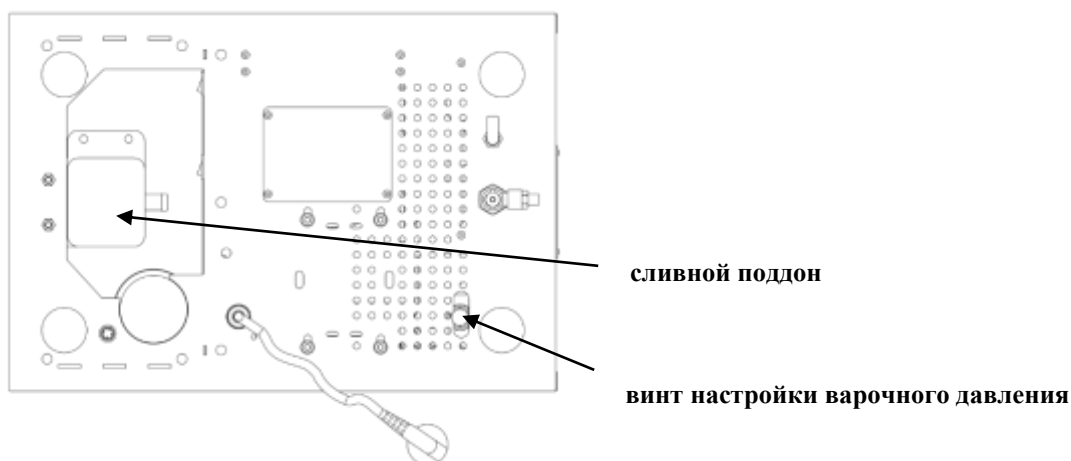
Рисунок 5: Дно машины
