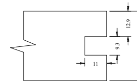
Moldura P-8mm
