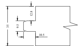
Respiga P-8mm
