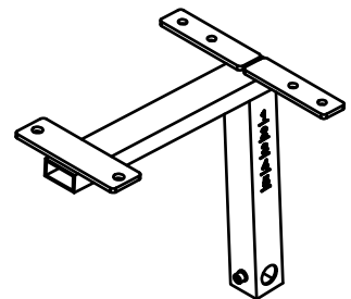
J[1PCS] 6650-001
