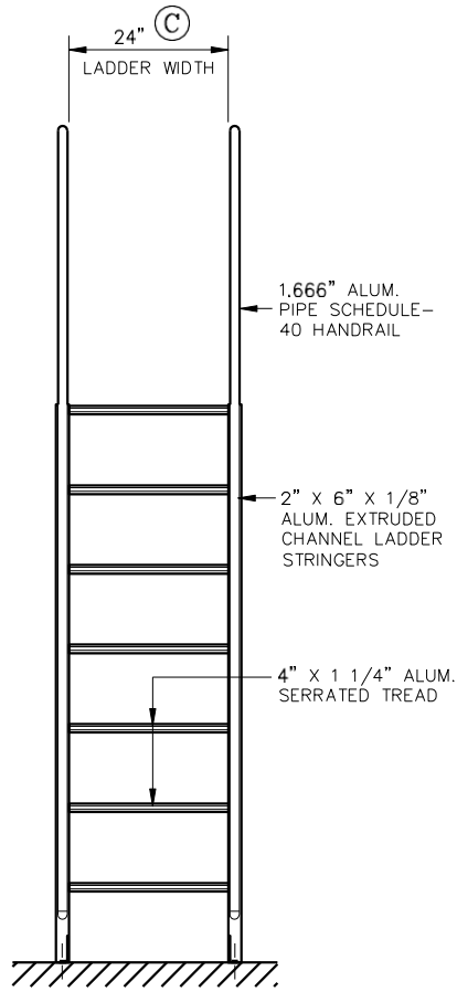
FRONT ELEVATION N.T.S.
