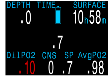
6. 희석 기체 점검
