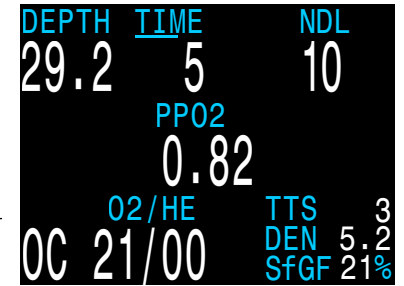
NDЛ 대체 미니 디스플레이 모습
