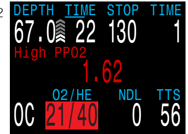
"High PPO2(PPO2 높음)" 고정 알림 예시
