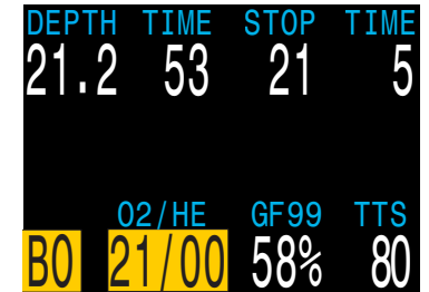
14. 기체 변경 필요
