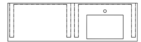
Right Bowl / Seno Derecha / Vasque Droite
