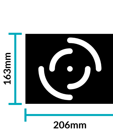
Baseplate
