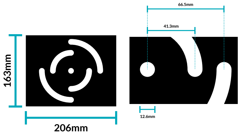
Baseplate
