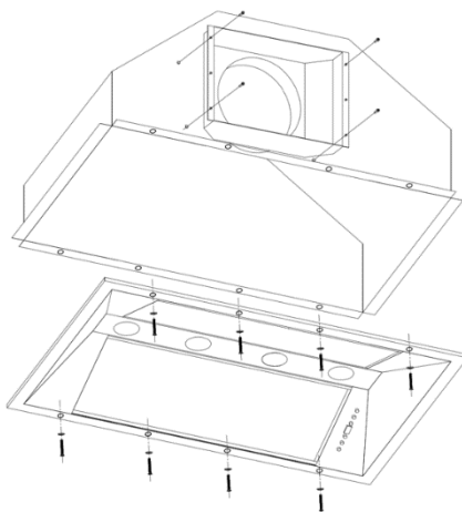
FRHRE5337-48
