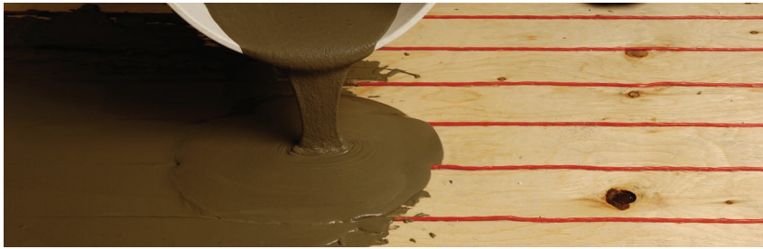
FIGURE 2.42 : Méthode du mélange autolissant
