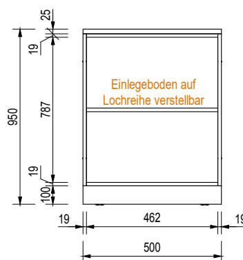
Ansicht Bedienseitig
