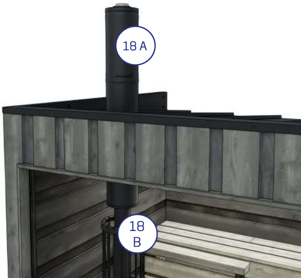
11. Pujota teräspiippu ( 18 A ) eristevillan ja katon lävitse. Laske teräspiippu savuputken ( 18 B.) päälle.
