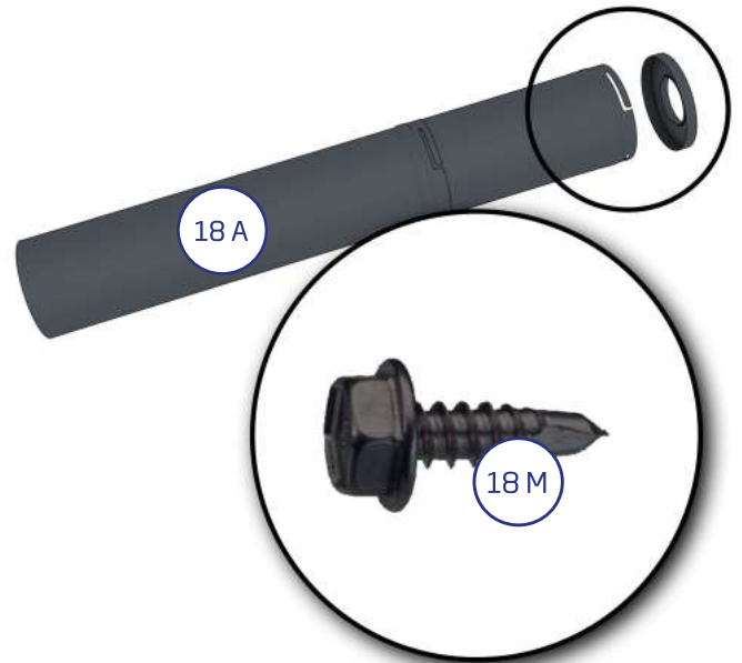
10. Kiinnitä yläpäätty teräspiippuun ( 18 A ) kolmella itseporautuvalla ruuvilla ( 18 M ). Ruuvit porataan pellin läpi.
