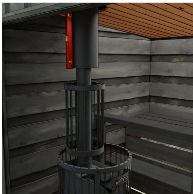
13. Vérifiez la rectitude de la cheminée. Déplacez le poêle si nécessaire.
